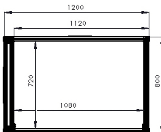
Schnitt Ebene 1
