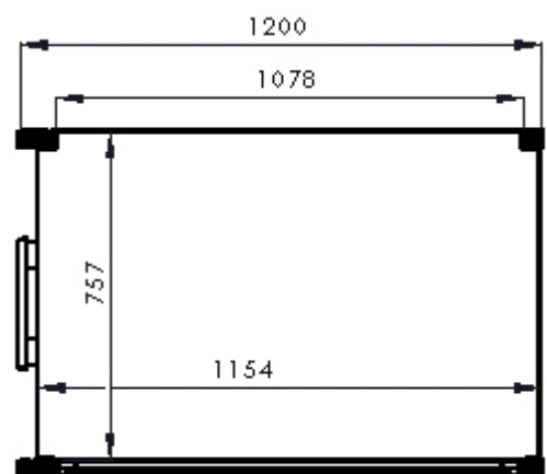
Schnitt Ebene 2
