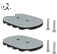
Bestell-Nr.: 019213 nivello®-Fußplatte für Gitterroste 126x89 mm
